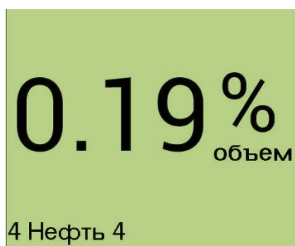
Рисунок 2 – Основное окно
