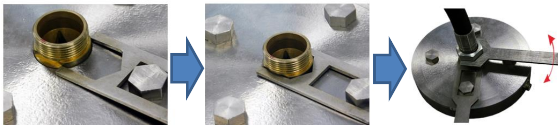
Рисунок 3 - Подключение РВД к первичному преобразователю
