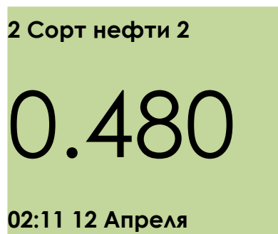
Рисунок 4 – Основное окно
