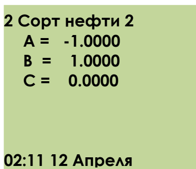
Рисунок 8 – Окно «Коэффициенты»
