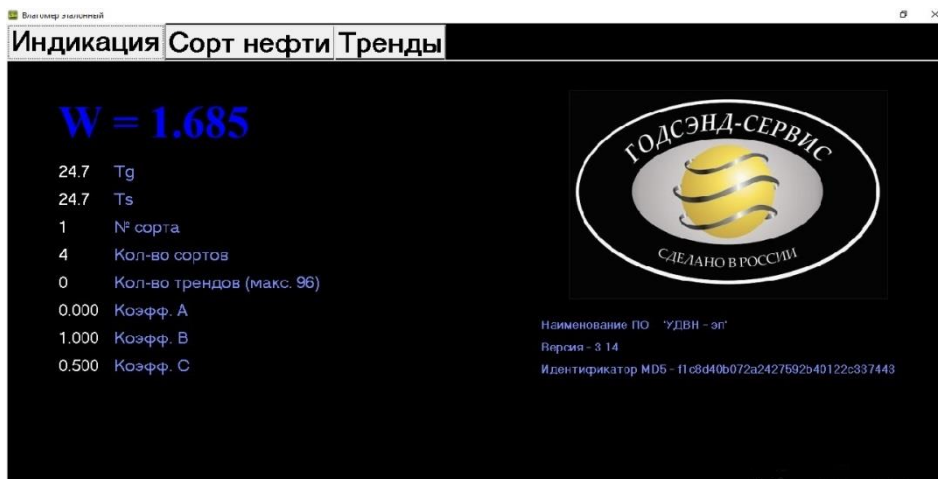
Рисунок 12 – Вкладка «Индикация»
