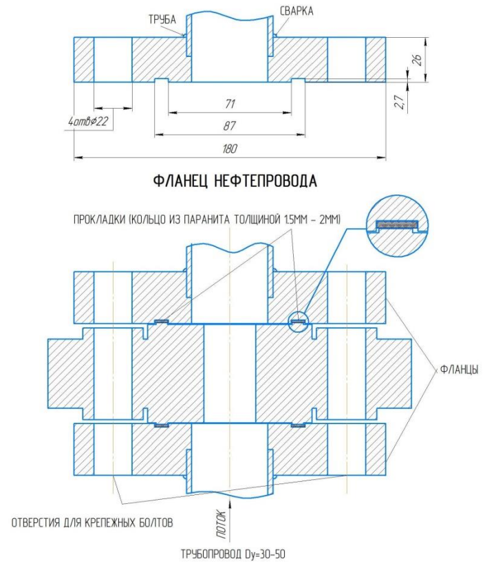
СХЕМА МОНТАЖА ПЕРВИЧНОГО ПРЕОБРАЗОВАТЕЛЯ
