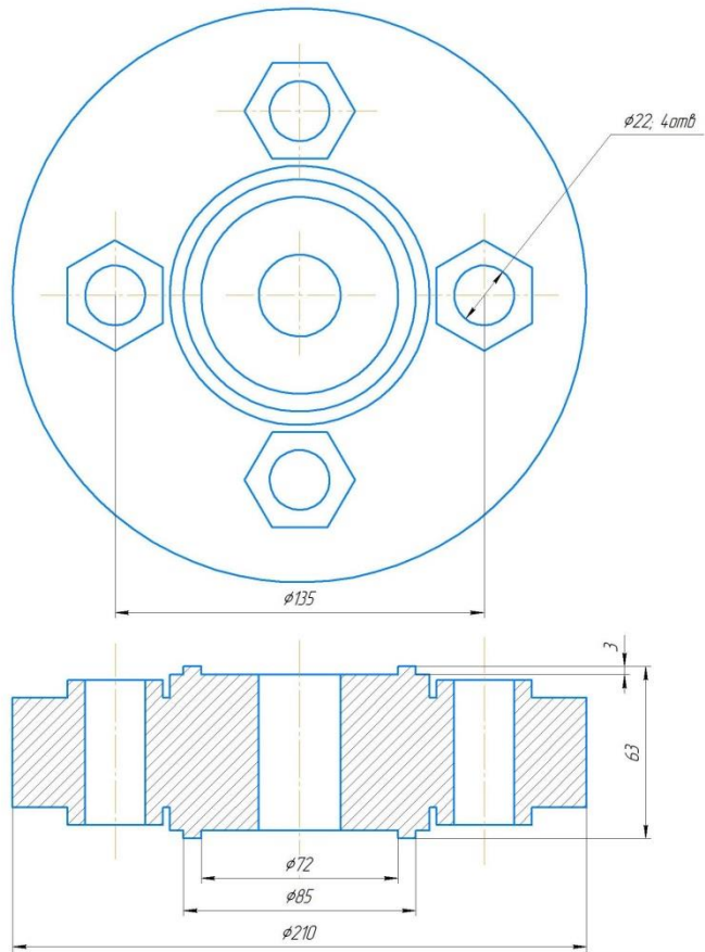
ПЕРВИЧНЫЙ ПРЕОБРАЗОВАТЕЛЬ
